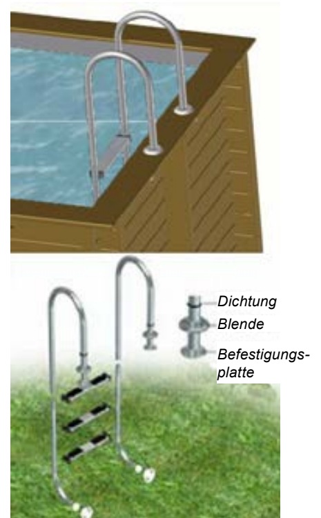
Abbildung 36 – Montage der Leiter
